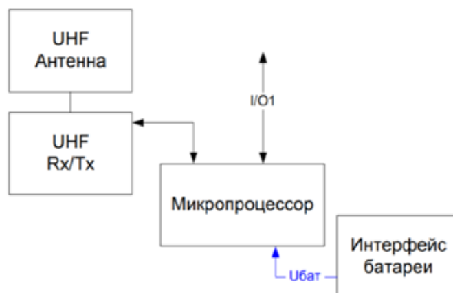
Блок-схема персонального транспондера IPT
